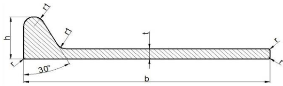
球扁钢的外形和尺寸示意图
